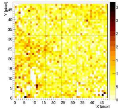
TLEs
